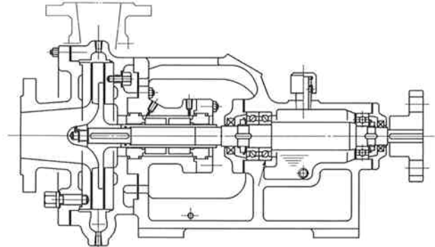
Double seal 図
